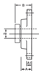
Side HCFT
