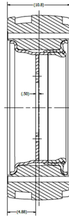
SECTION A-A
