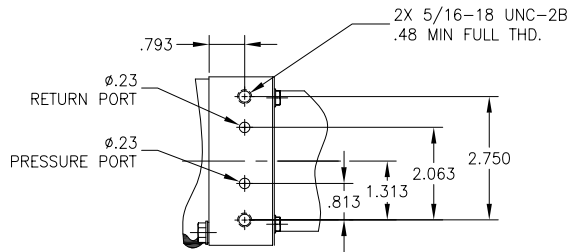
VIEW A-A
