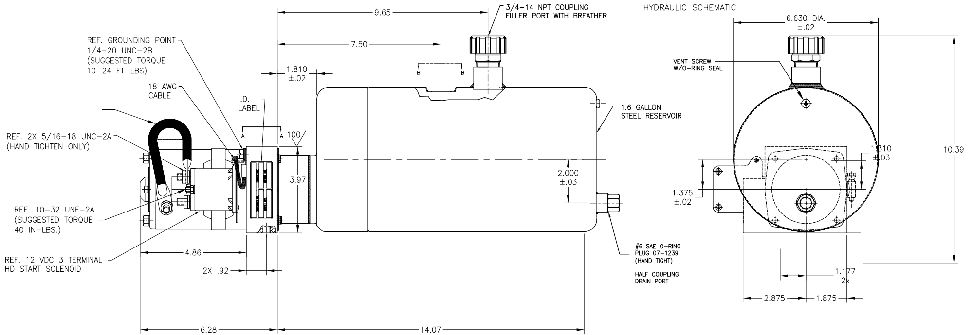
VIEW A-A
